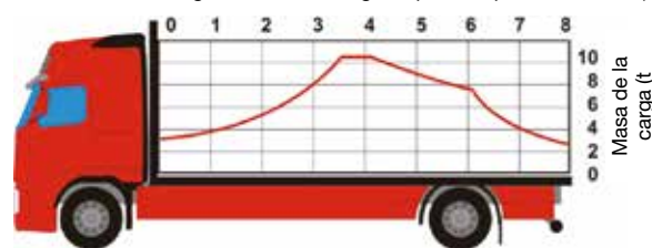
Fig. 2. Ejemplo de diagrama de distribución de masas – vehículo motorizado de dos ejes.
