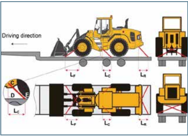
Fig. 31. Fijación directa.
